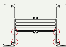
・屋内型 (施工時に接続カバーも防水コーキング)
