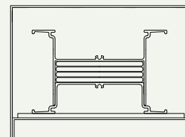
・屋外型 (外箱+防水コーキング)
